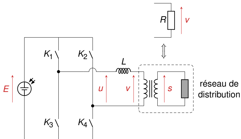
FIGURE 1 – Schéma de principe de l'installation électrique.
