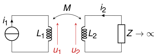
FIGURE 5 – Schéma électrique équivalent du transformateur.
