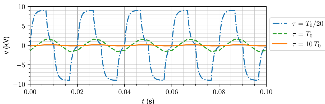
FIGURE 3 – Tension lissée v en fonction du temps.
