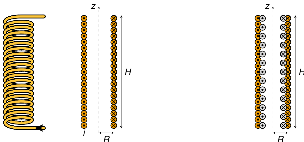
FIGURE 4 – Modélisation du transformateur. Gauche : schéma d'un solénoïde unique. Droite : modélisation du transformateur par deux solénoïdes imbriqués.
