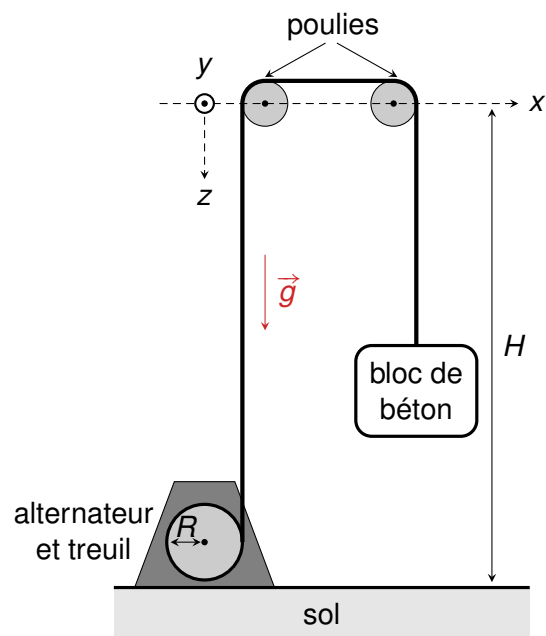
FIGURE 6 – Démonstrateur Gravitricity.
